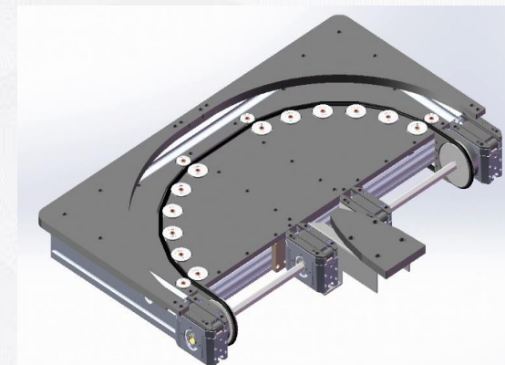
KE 2/180 Curve KE 2/180 弯道
