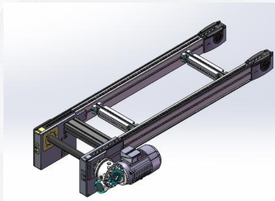
UTS2 ARC2-H Roller Chain Conveyor UTS2 重载滚子链输送线
