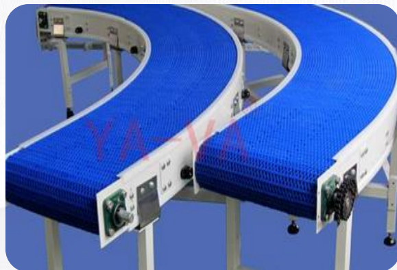
直/转弯塑料网带输送线 塑料网格/输送线
