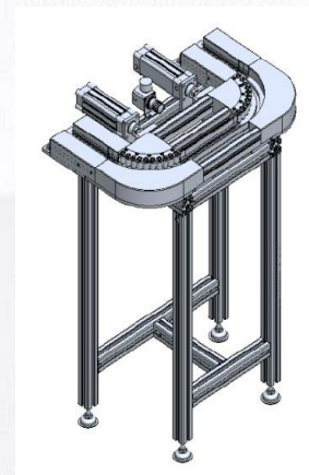
Tension Unit 张紧单元
