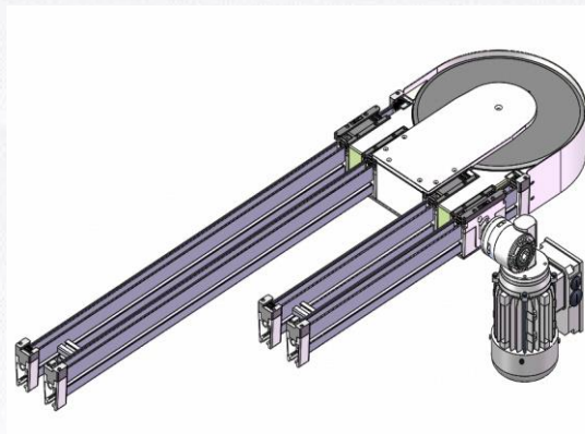
180° Curve 180°圆盘转弯
