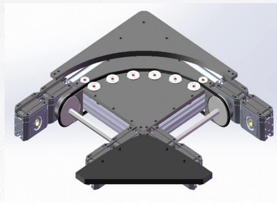
KE 2/90 Curve KE 2/90 弯道
