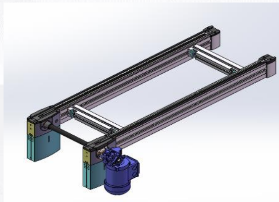
UTS2 ARC2 Roller Chain Conveyor UTS2 轻载滚子链输送线
