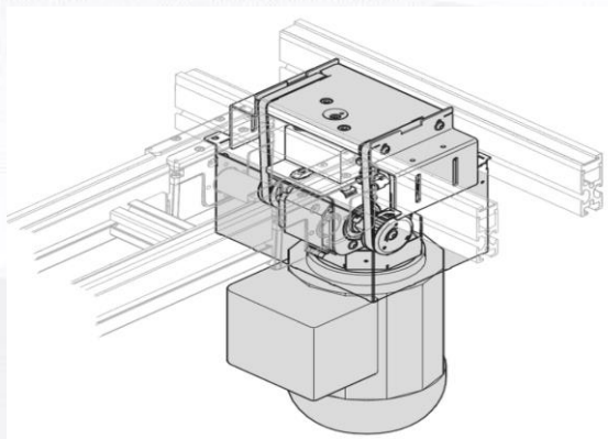
Lifer Transfer Unit 顶升横移单元
