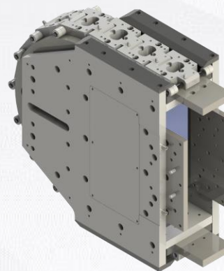
DMETU End Tension Unit 尾部张紧单元
