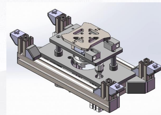
Lift Rotate Unit 2 顶升旋转单元
