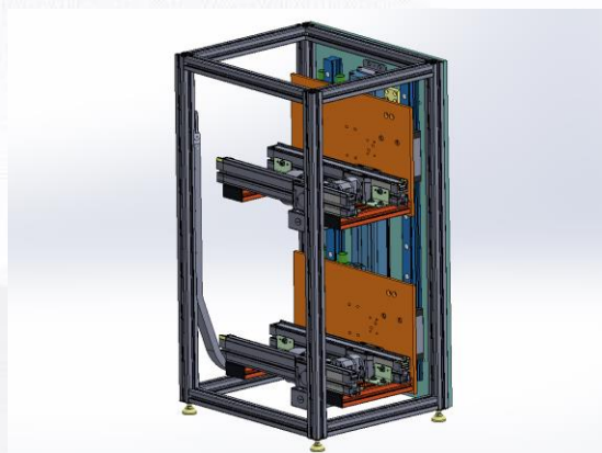
Lift Unit 2 提升机
