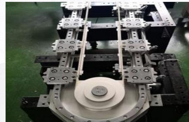
环形导轨输送线 蜗轮蜗杆/同步带
