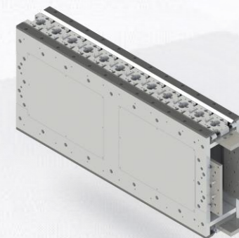
960mm Middle Unit 960mm 中间线体
