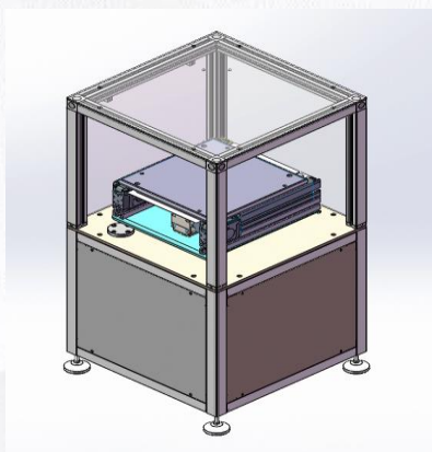
Rotate Unit 2 旋转台
